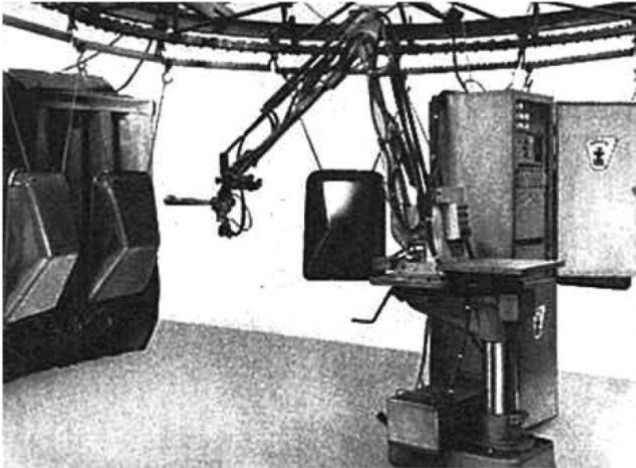
Robô para pintura automática de veículos 1965-7 – Trallfa (Noruega)
